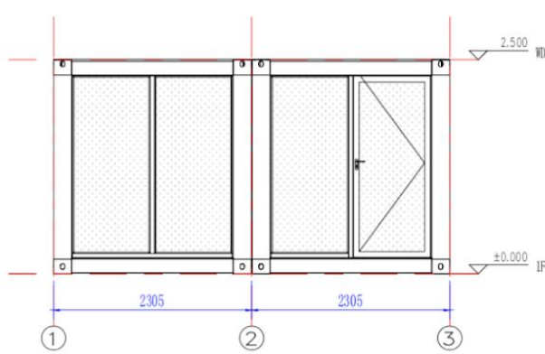
Vista Frontale
